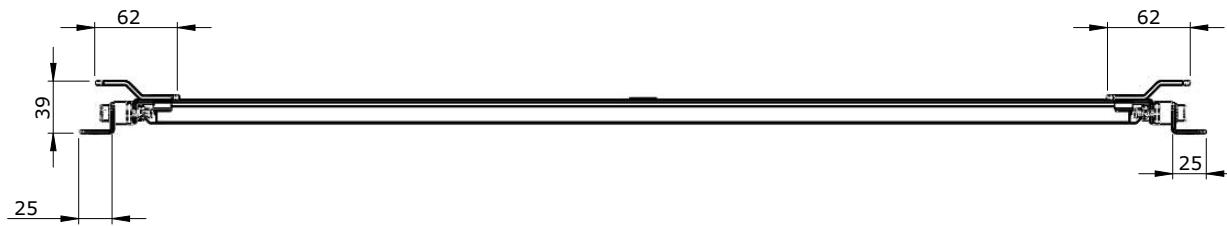
SECTION A-A SCALE 1 : 4
