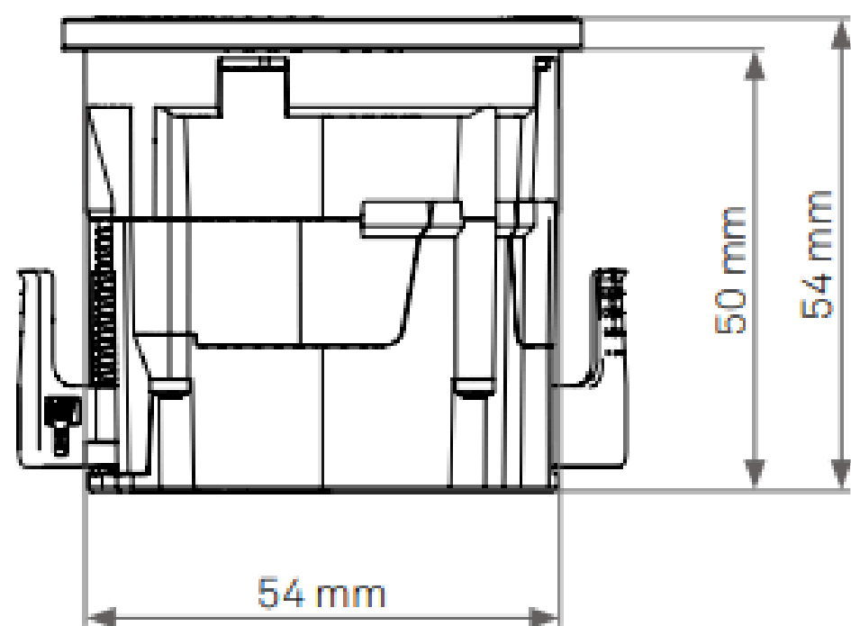
Klemmstück Clamp
